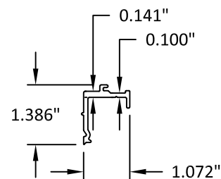
11 FLUSH FILLER
